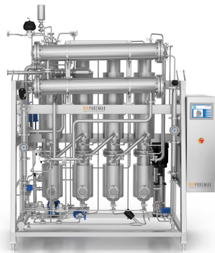
Destilador de Multiefeito
